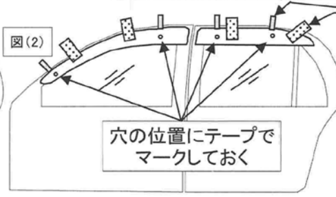
図(1) 窓ガラスを下げてランチャンネルを図のように外す
